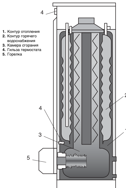
Рис. 15: Конструкция котла
