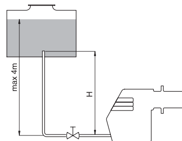
Рис. 8а: Схема без термостатического смесителя.
