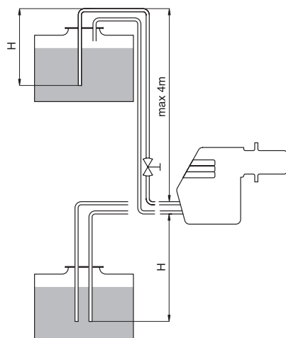
Рис. 8б: Питание топливом с обратной магистралью при высоко или низко расположенном баке
